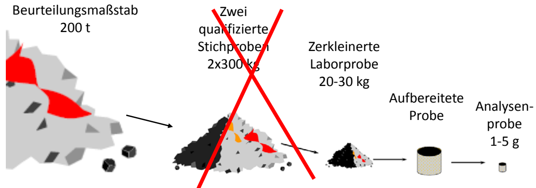
Abbildung 8: Bei der Direkten Ballenbeprobung fällt bei der Probenahme ein Aufbereitungsschritt weg.
