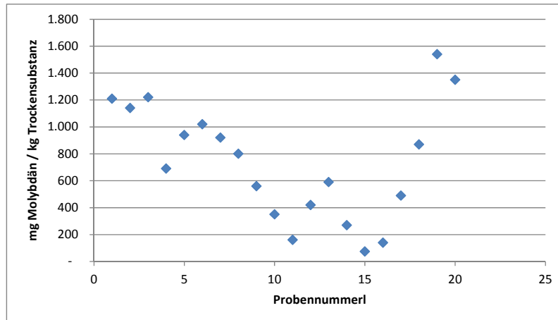
Abbildung 4: Molybdänkonzentration in 20 Stichproben, die nach dem Stand der Technik entnommen wurden (nach der Zerkleinerung auf 30 mm).
